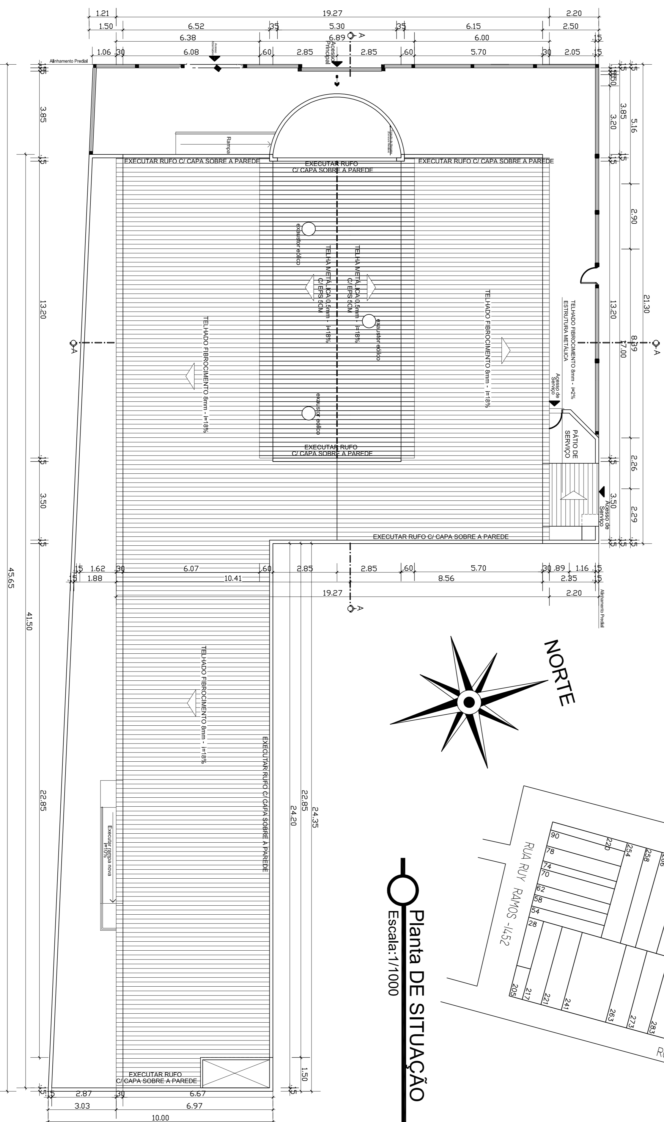
Planta Cobertura e Localização Escala: 1/100
