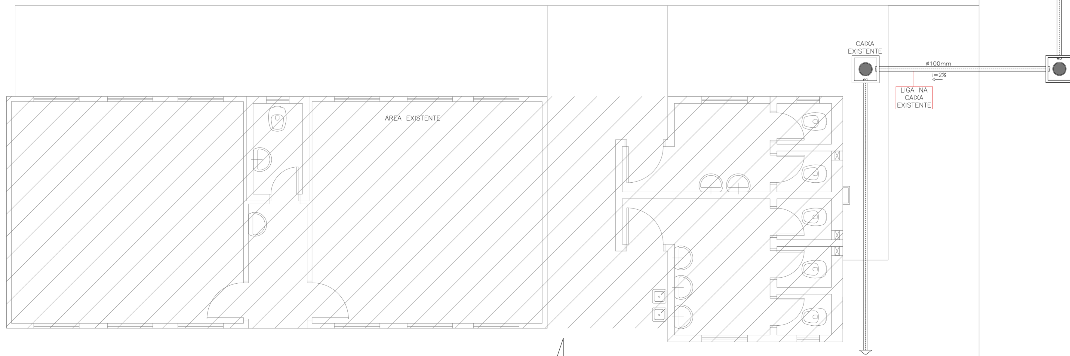
PLANTA SANITÁRIA ESC. 1:50
