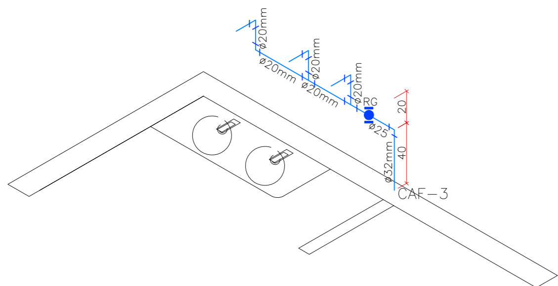
ESTEREOGRAMA LAVATÓRIOS E EBBEDOURO LAVATÓRIOS E BEBEDOURO REFEITÓRIO ESC. 1:25
