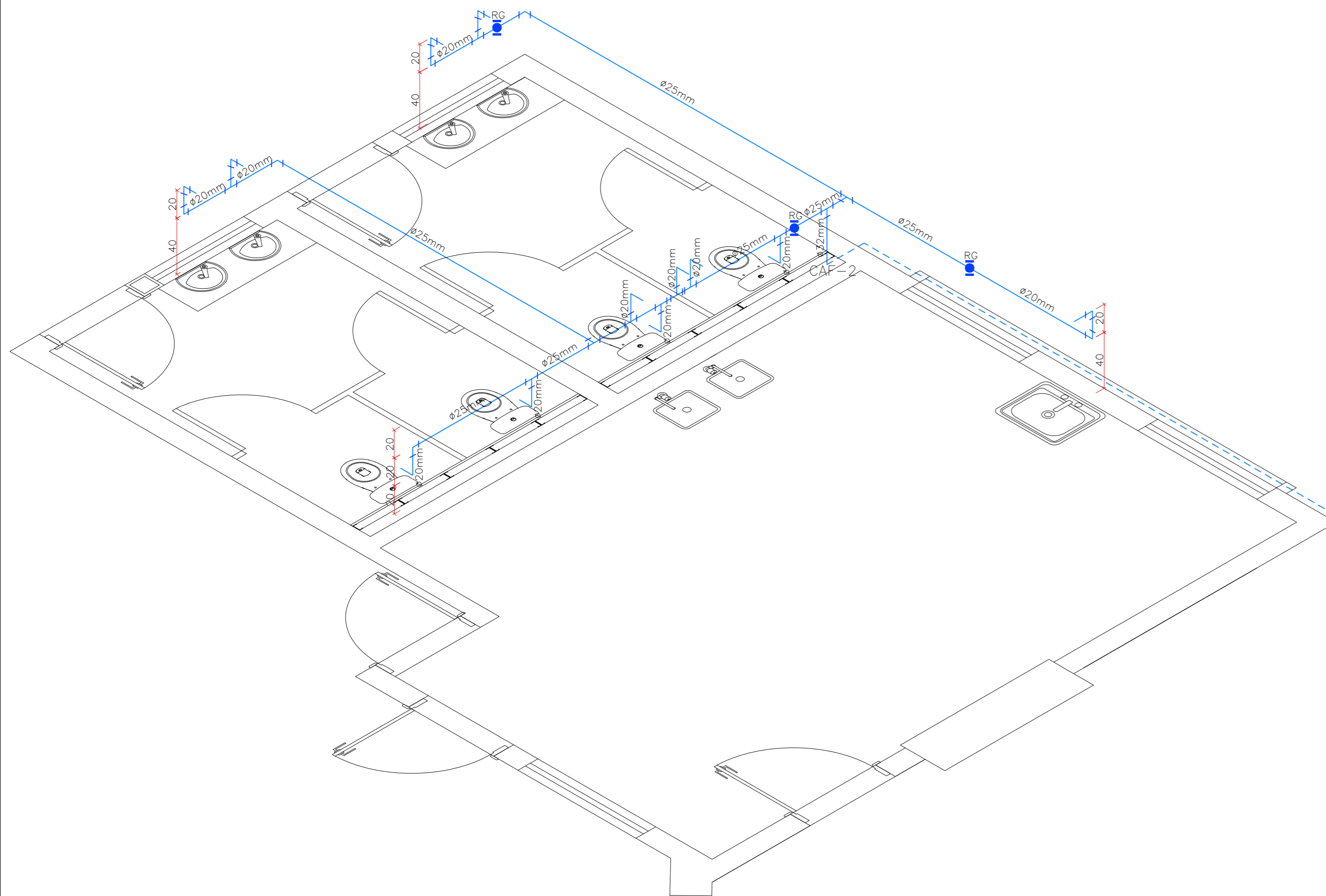
ESTEREOGRAMA COZINHA E WC ESC. 1:25
