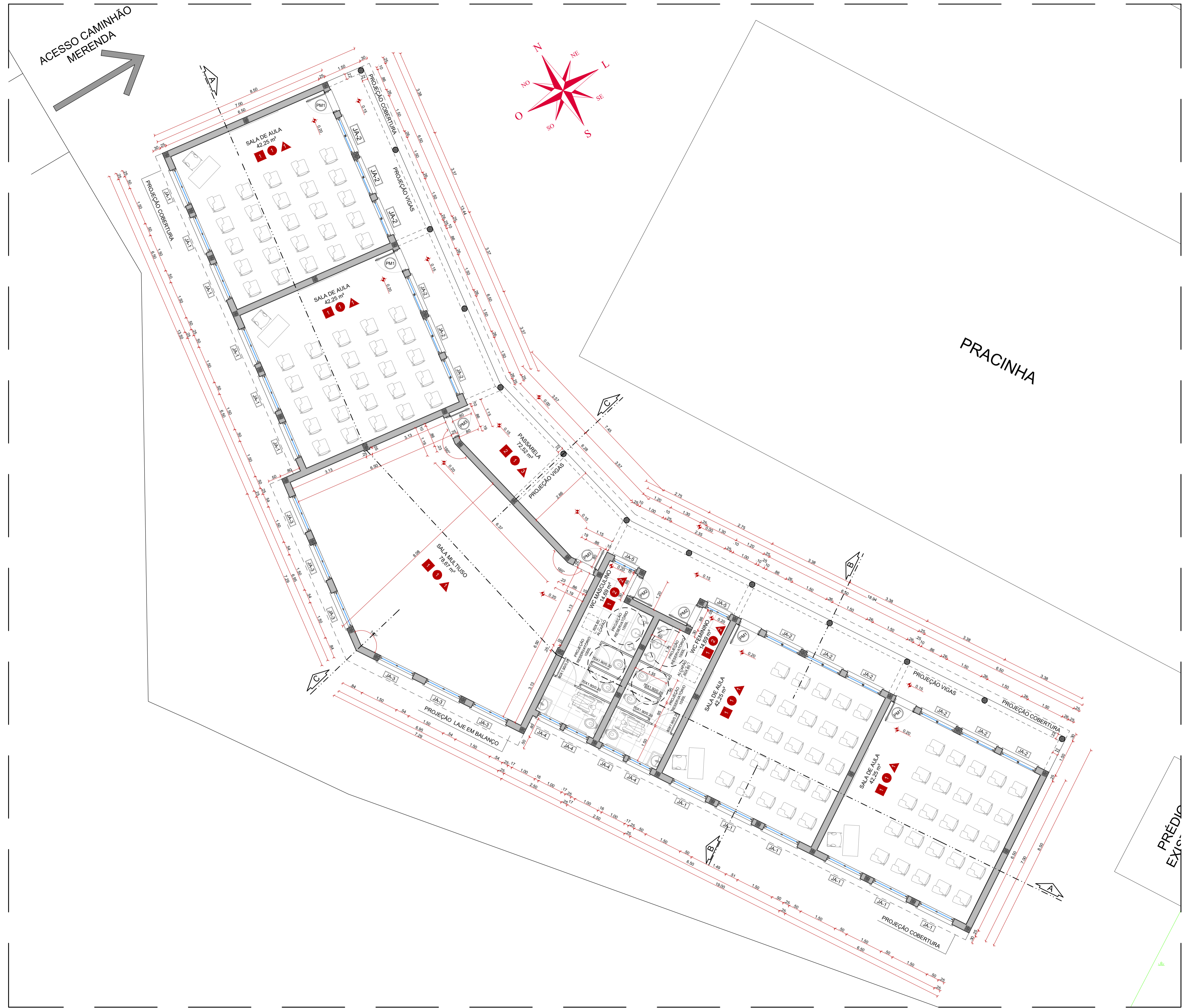
01 PLANTA BAIXA ESCALA 1/75
