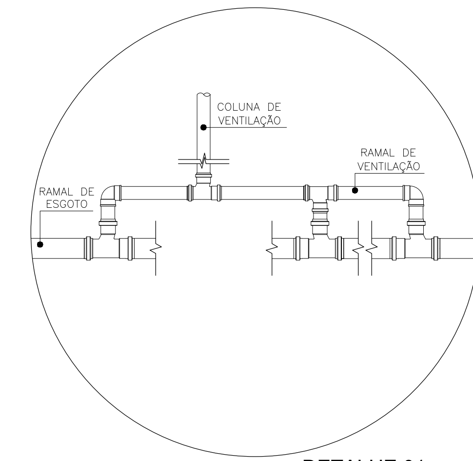
DETALHE 01 ESQUEMA DE LIGAÇÃO DO RAMAL DE VENTILAÇÃO ESC. 1:20
